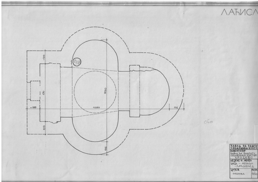
Сл. 11. Локалитет Црквина у Лаћиследу, основа цркве (Документација Завода за заштиту споменика културе Краљево)
