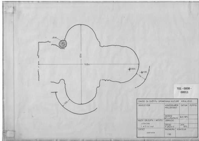
Сл. 2. Локалитет Црквина у Лаћиследу, ситуациони план основе цркве пре почетка археолошких истраживања 1972. године (Документација Завода за заштиту споменика културе Краљево)
