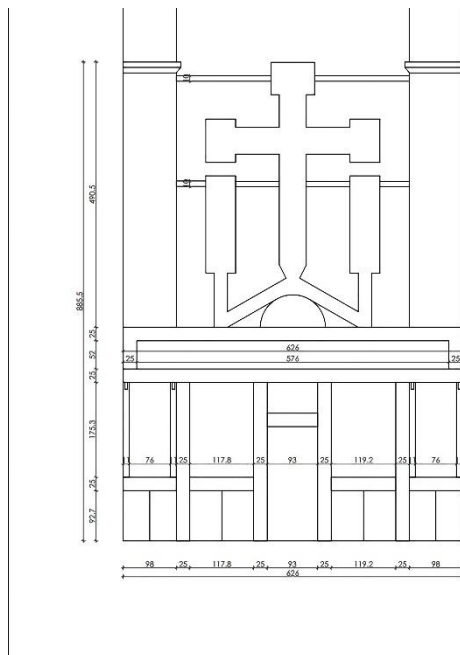
Сл. 4. Реконструкција сопоћанског иконостаса са kotaма (Исидора Кисин, Урош Марковић)
